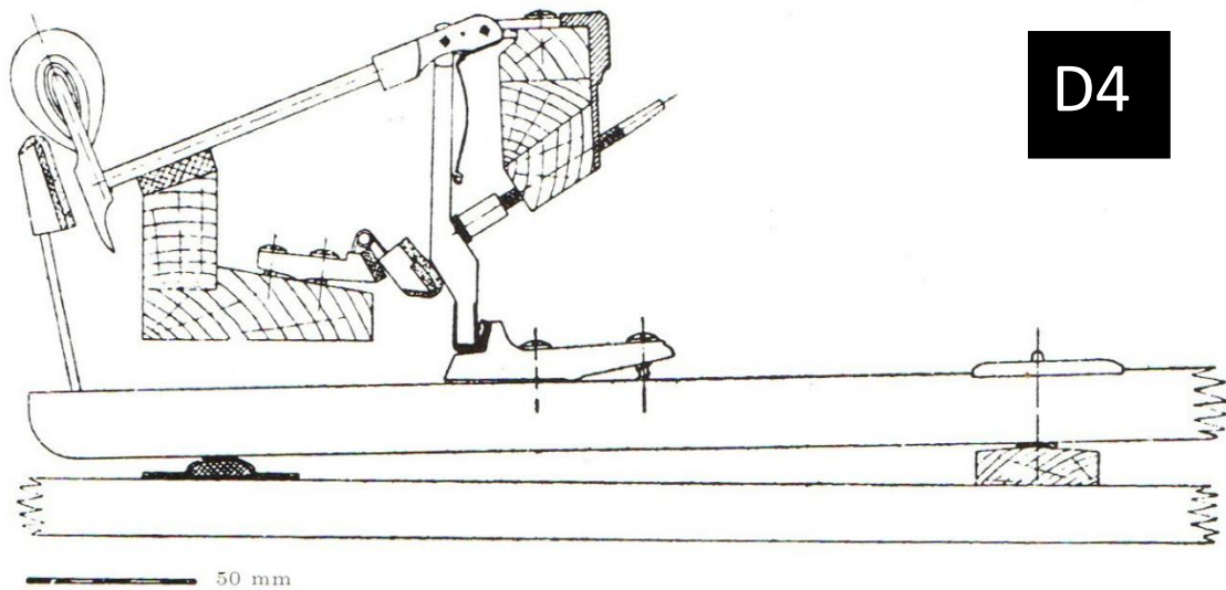
FIG. 47 – Mécanique articulée, bâton à pivot inversé. Herrburger-Schwander, Paris. Milieu du XIX e siècle environ. Musée de Stuttgart.
