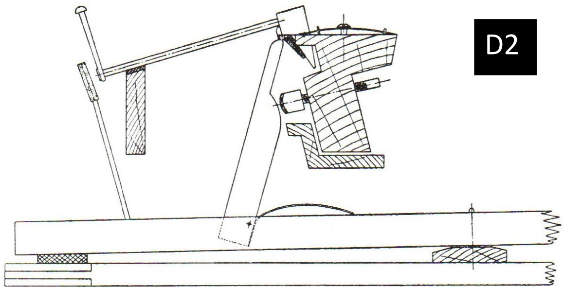
FIG. 29 – Forme la plus ancienne du bâton à surface glissante. Robert Stodart, 1777. D'après le brevet anglais.
