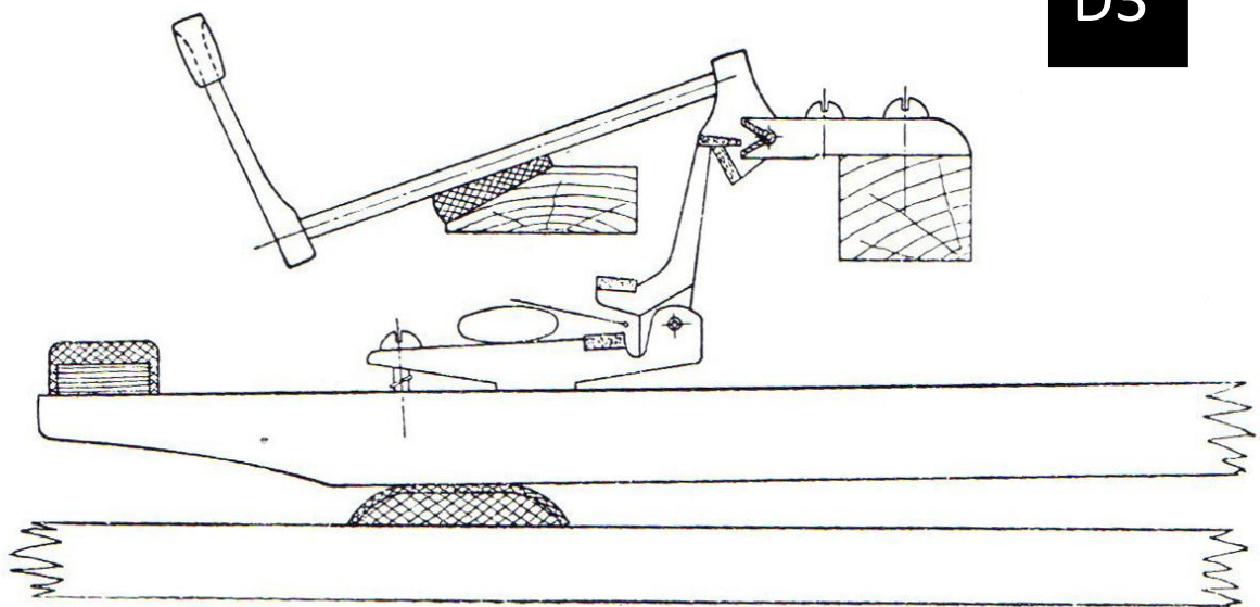
FIG. 30 – Bâton en équerre de Petzold. Environ 1810. D'après Rosamond Harding.
